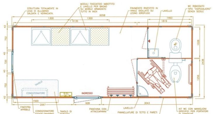
Grundrißdarstellung der Einheit in operativem Zustand mit Standardausstattung
