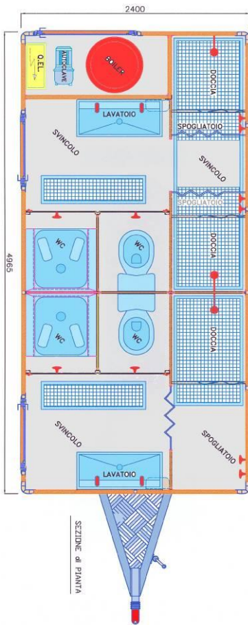
Vista/plano de planta del conjunto
