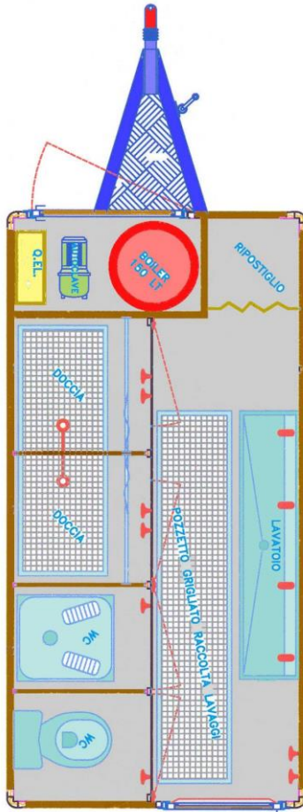
Vista/plano de planta del conjunto
