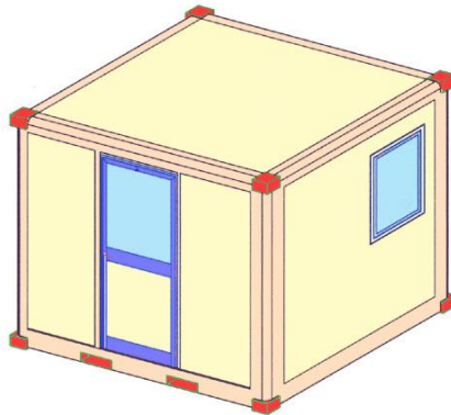
Gesamtansicht in "geschlossener" Position (Standard ISO-10')
