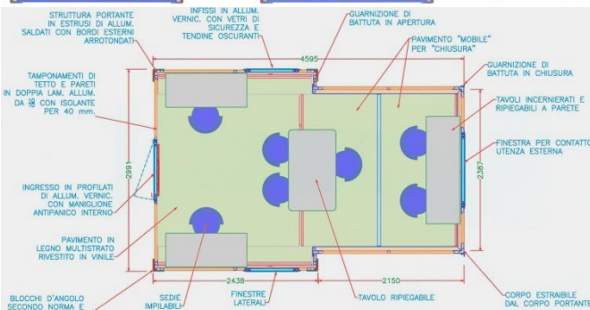
Grundriss in betriebsbereiter Position
