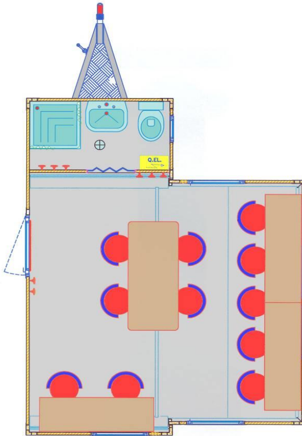
Vista/dibujo en planta del conjunto "extendido" en posición operativa
