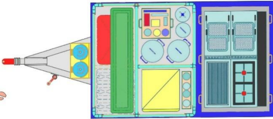
Grundrissdarstellung der ausgestatteten Shelter Anlage + Küchenblock
