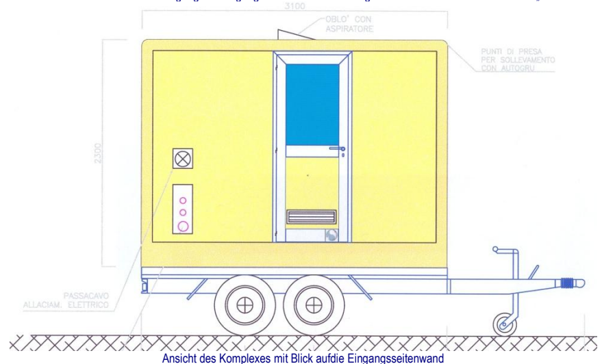
Ansicht des Komplexes mit Blick auf die Eingangsseitenwand
