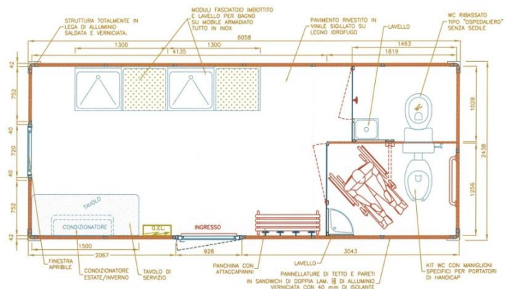
Vista in pianta del complesso in formazione operativa con allestimento standard
